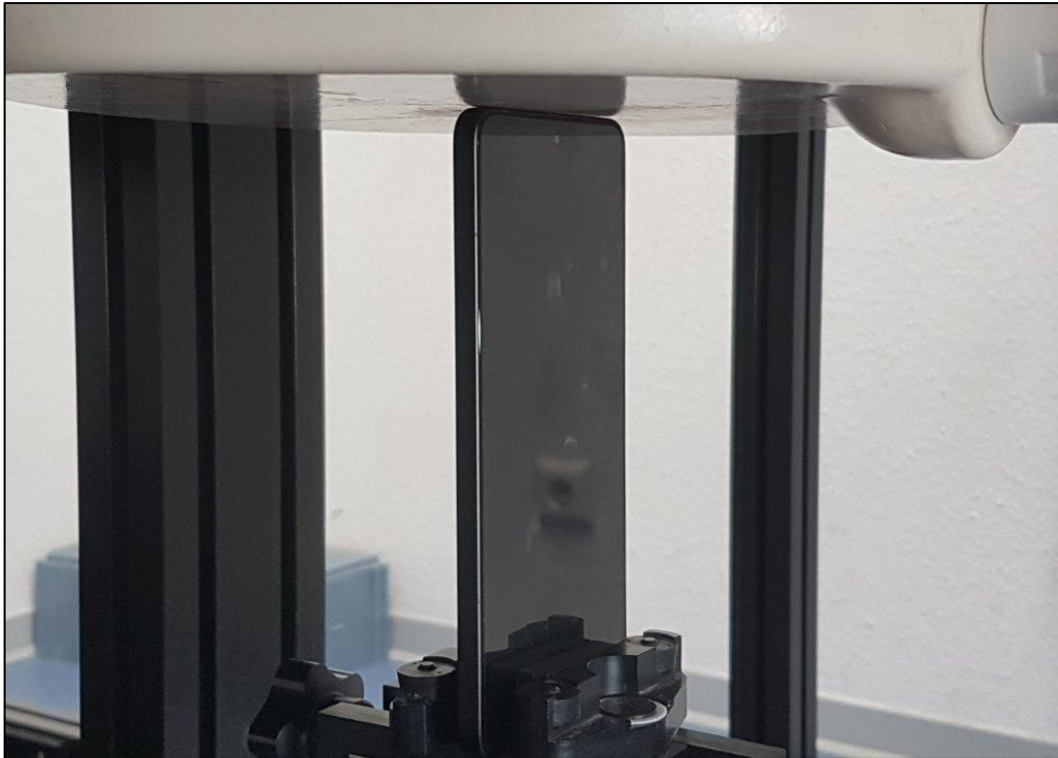
Photo 12: Position d'essai face du dessous contre le membre (distance 0 mm)
