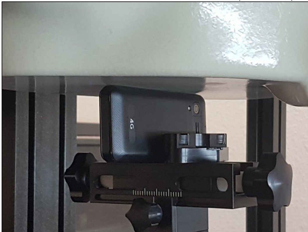
Photo 12: Position d'essai face du côté droite contre le membre (distance 0 mm)
