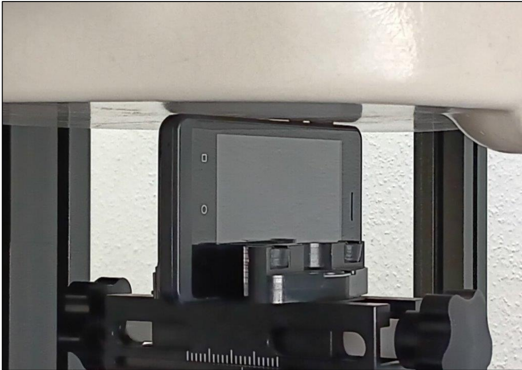
Photo 12: Position d'essai face du côté droite contre le membre (distance 0 mm)
