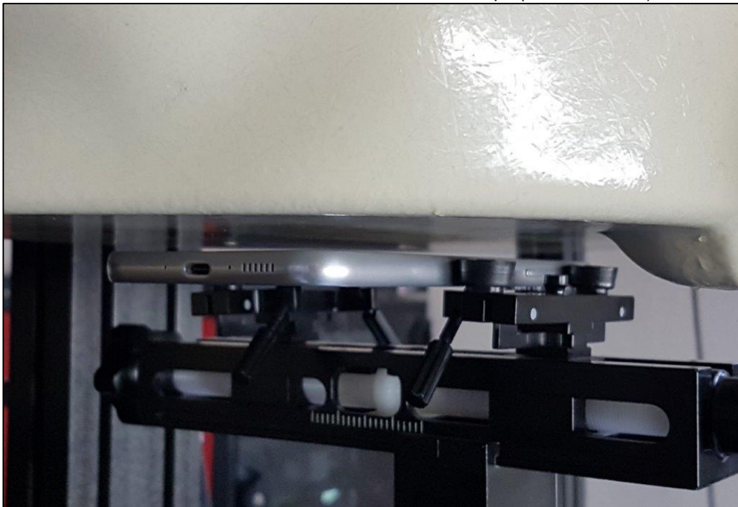
Photo 8: Position d'essai face arrière contre le corps (distance 5 mm)
