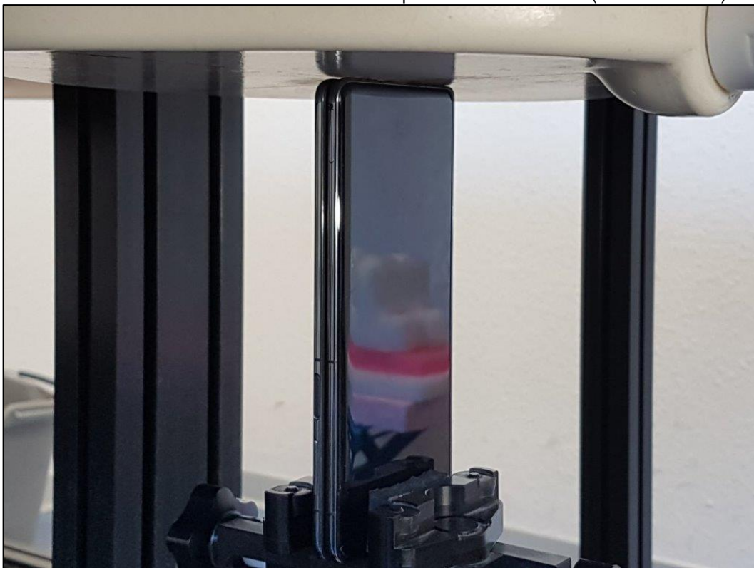
Photo 13: Position d'essai face du dessous pilé contre le membre (distance 0 mm)
