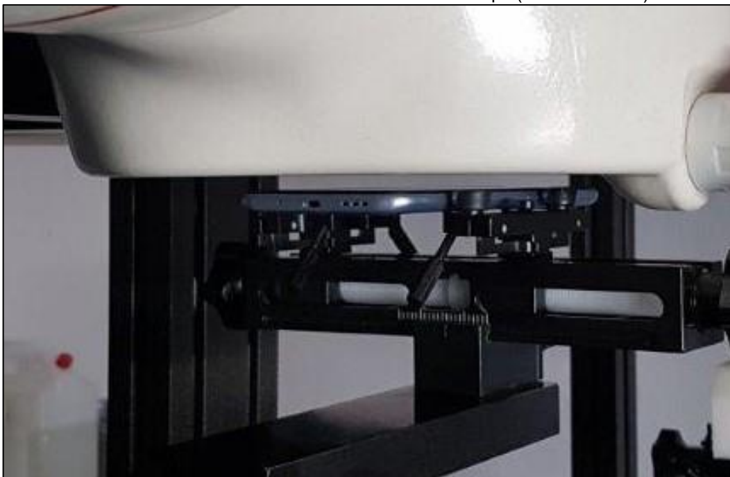
Photo 7: Position d'essai face avant contre le corps (distance 5 mm)
