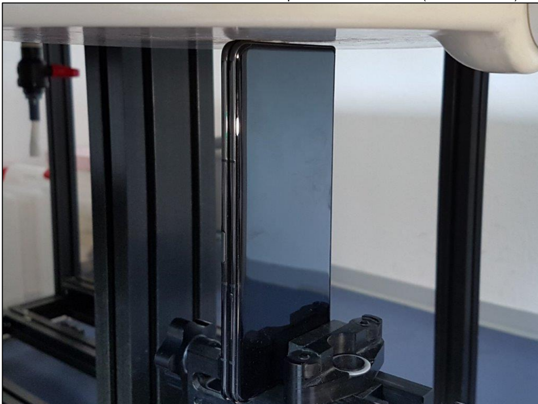
Photo 17: Position d'essai face du dessous plié contre le membre (distance 0 mm)
